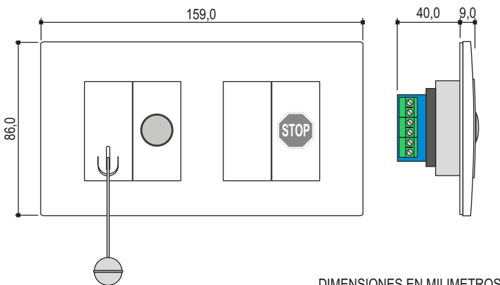
DIMENSIONES EN MILIMETROS
